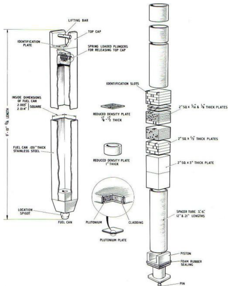
Fig. 5: 臨界実験装置 ZEBRA における燃料要素
