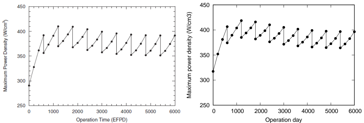
Fig. 13: 最大出力密度の比較 (左: 文献より引用、右: CBZ)
