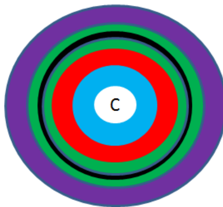
Fig. 11: 円筒状にモデル化された高速炉心
