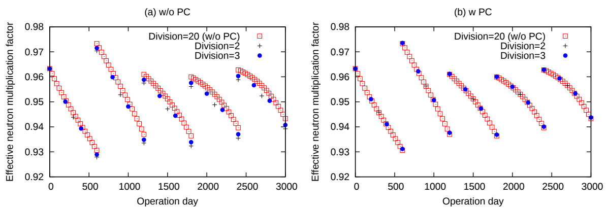
Fig. 16: 中性子実効増倍率の燃焼ステップ分割数に対する依存性（予測子-修正子法の効果）
