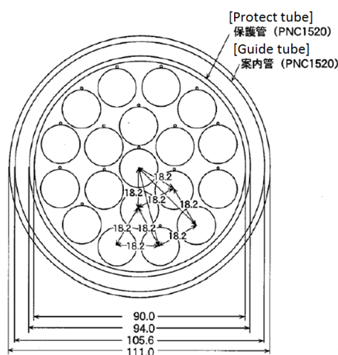
Fig. 5: 「もんじゅ」制御棒の形状
