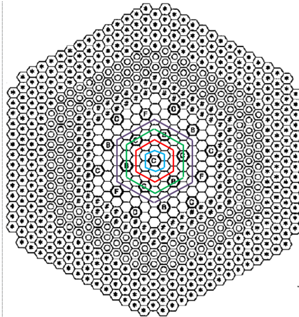
Fig. 10: 円筒にモデル化する高速炉心
