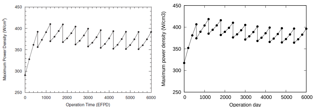
Fig. 14: 最大出力密度の比較 (左: 文献より引用、右: CBZ)
