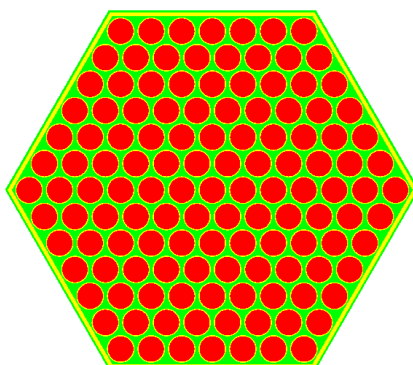
Fig. 4: CLIP による燃料集合体の図示の例
