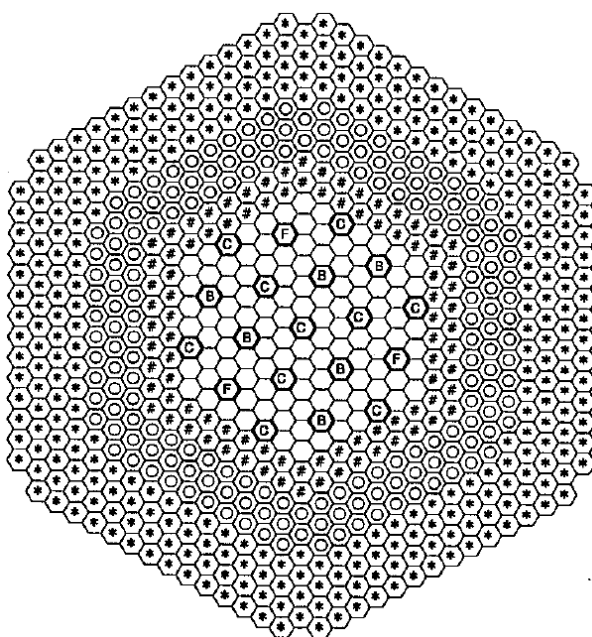
Fig. 7: 中型高速増殖炉の燃料配置図
