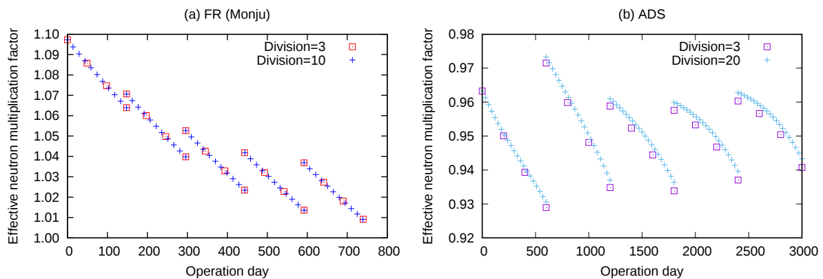
Fig. 15: 中性子実効増倍率の燃焼ステップ分割数に対する依存性
