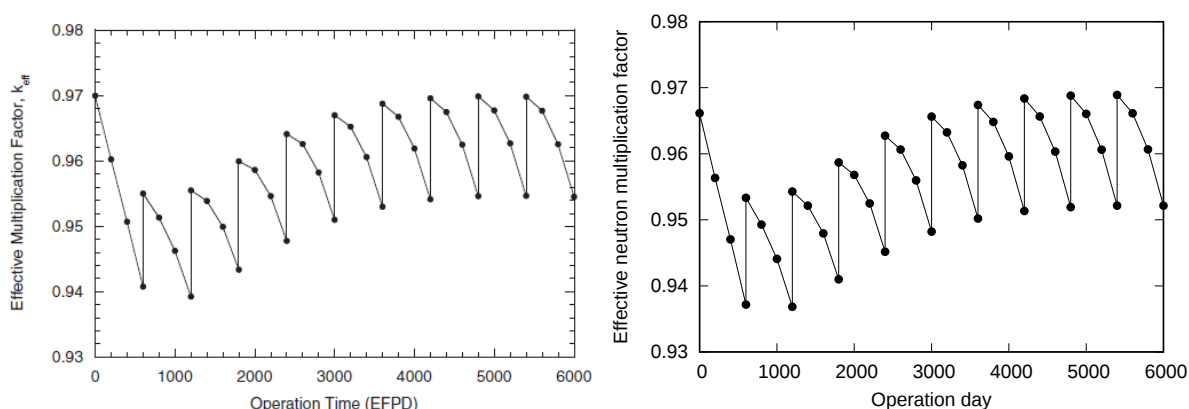
Fig. 13: 中性子実効増倍率の比較 (左: 文献より引用、右: CBZ)
