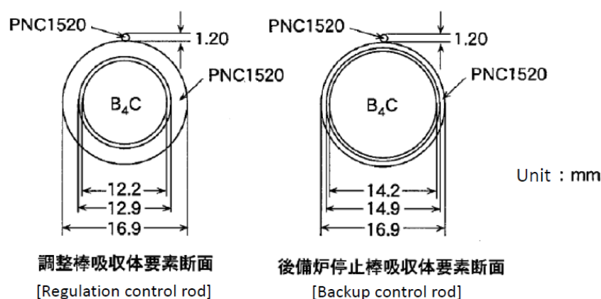
Fig. 6: 「もんじゅ」制御棒の吸収ピンの構造
