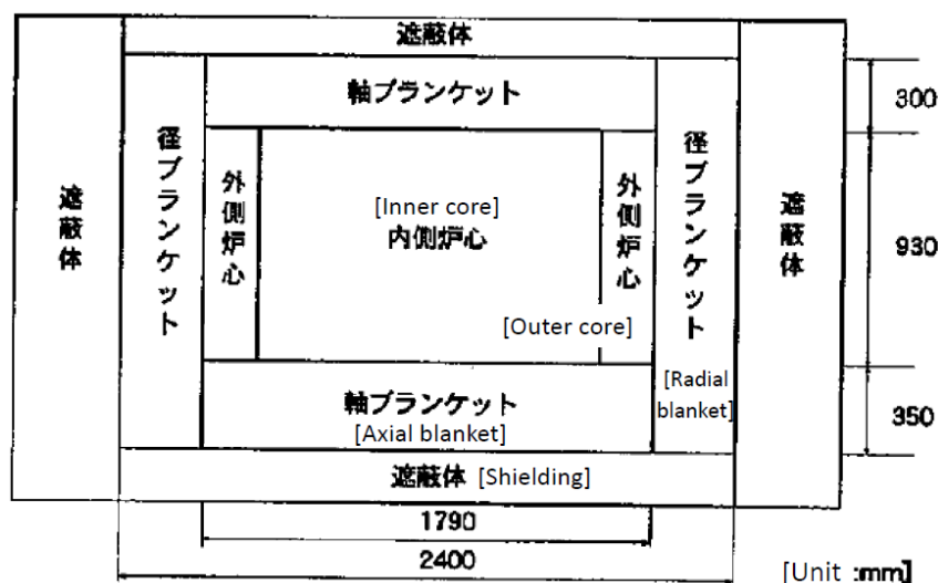
Fig. 8: 中型高速増殖炉の円筒モデル
